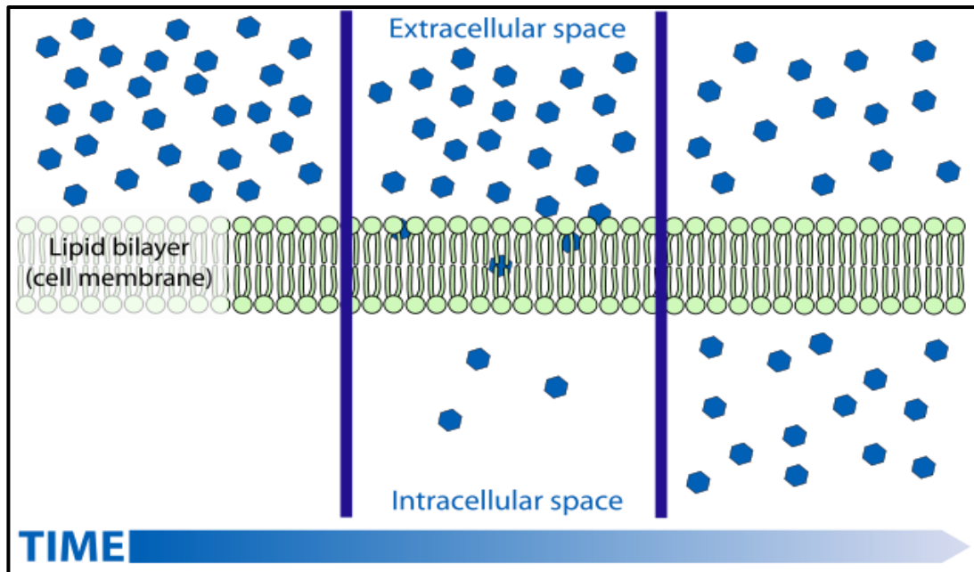
Figure 2: Simple diffusion
