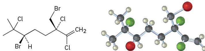
Halomon
