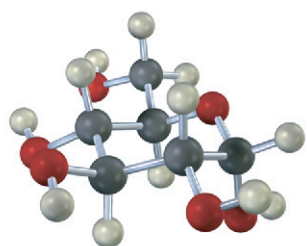
\alpha -Glucose
