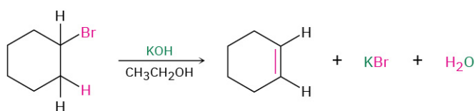
Bromocyclohexane
