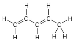
1,3-Pentadiene
