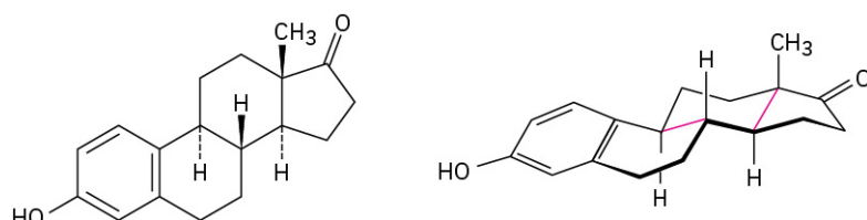
Estrone
