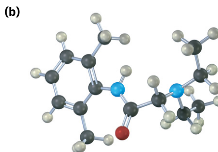
Lidocaine
