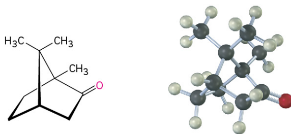
Camphor
