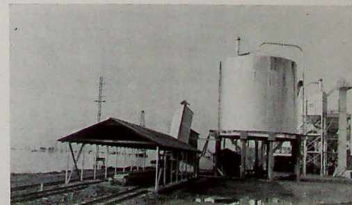
Gusano conductor de sacos y tanque para cemento.
