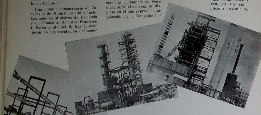
De izquierda a derecha, alambiques y fraccionadores, tuberías de aire y vapor, torres de absorción y estabilización, y otra vista de los alambiques y fraccionadores.
