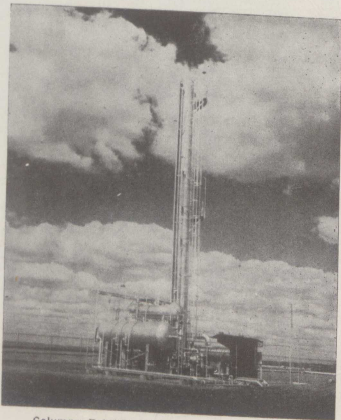
Columna Estabilizadora de gasolina natural.
