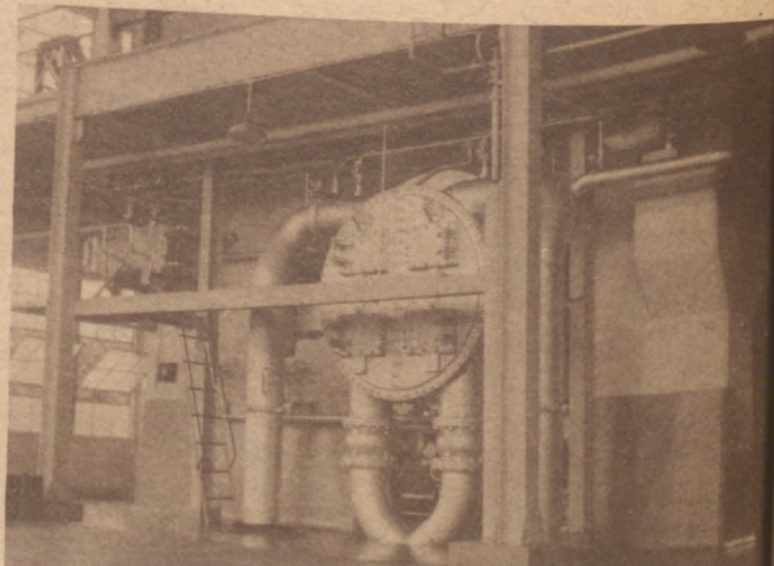
Nuevo condensador en la Planta de Las Morochas.
