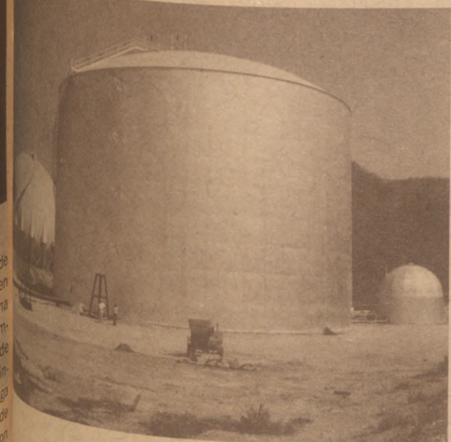
Tercer depósito de gas licuado de 120.000 bl.
